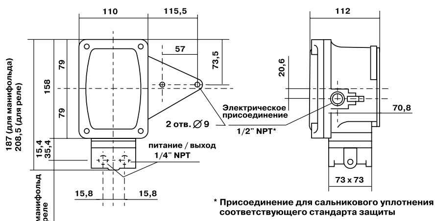
Рис. 3. Размеры, мм
