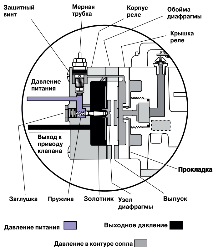
Рис. 2. Реле
