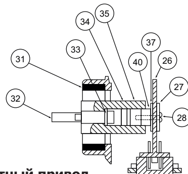
Поворотный привод
