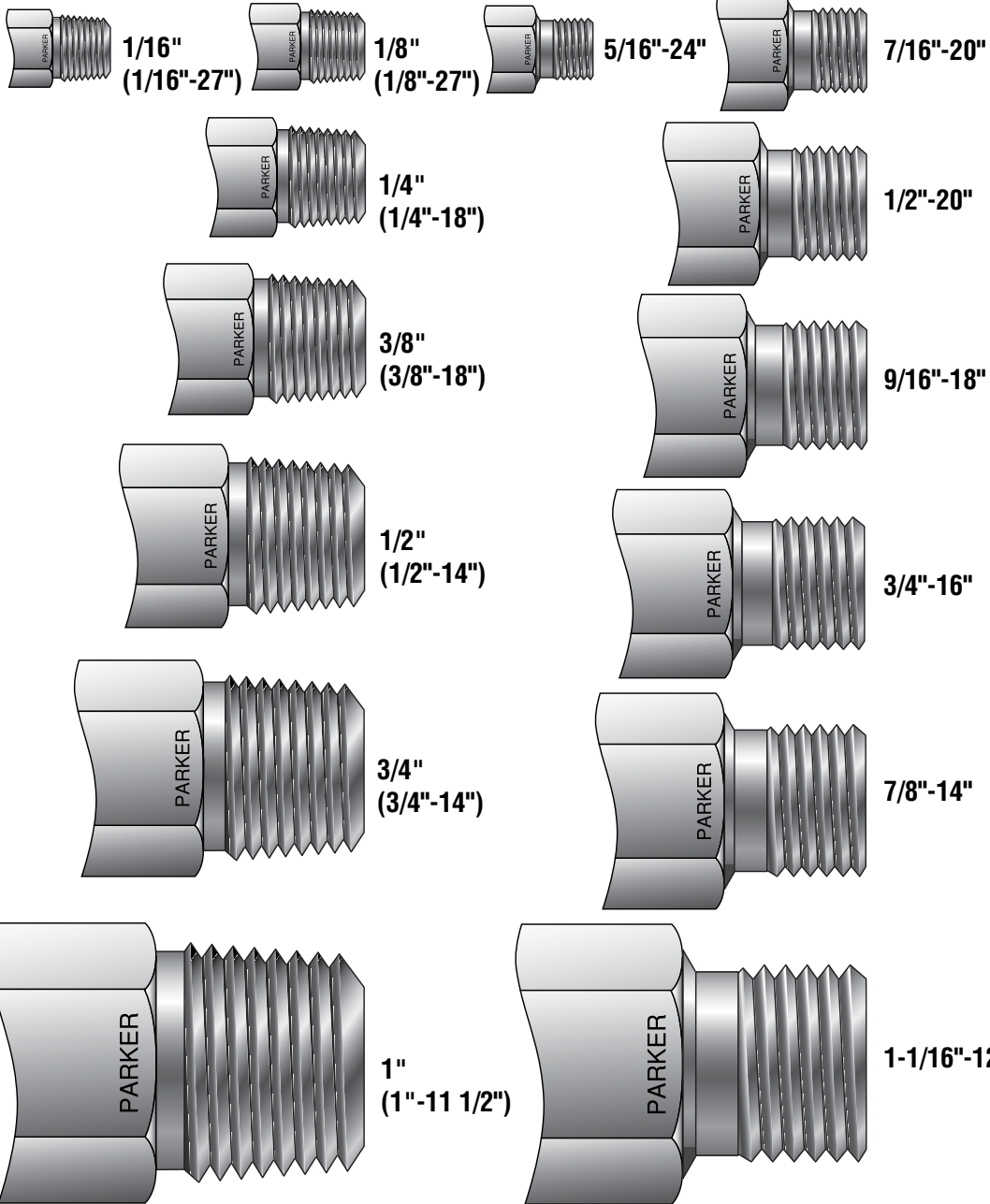
Стандарт США Резьба трубы (норм. трубная резьба)
