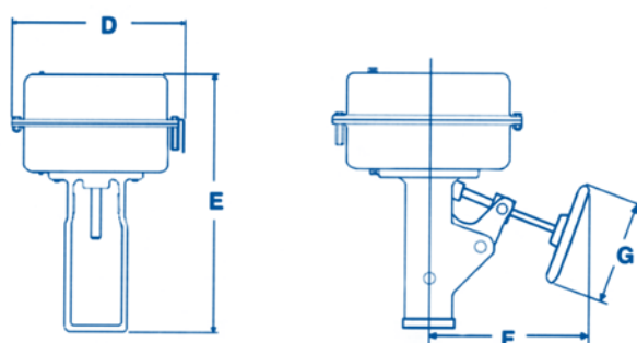
Привод серии 87/88 (ручной дублер – опция)
