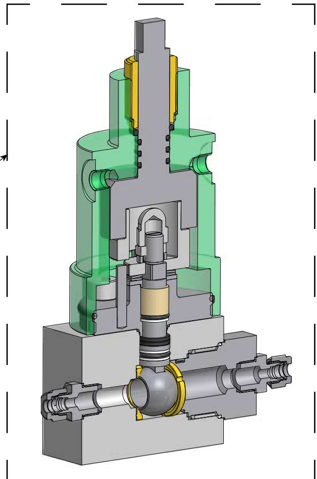
Шаровой клапан ISO 15848-1 Сборочный узел для испытания прототипа
